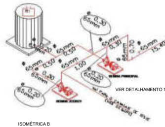
ISOMÉTRICA B SEM ESCALA
